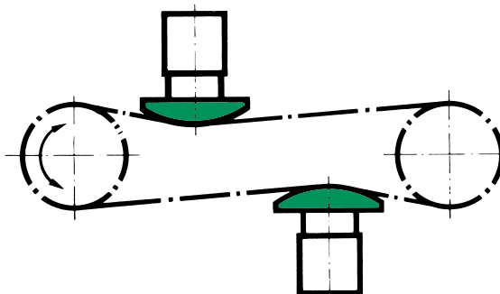
4. Olika placering av NONFRIC® SPÄNNBOX
