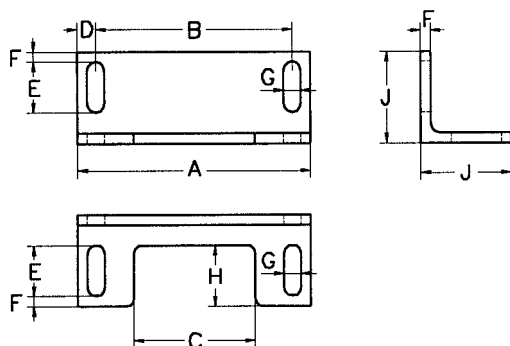
Fästvinkel för storlek 1 och 2
